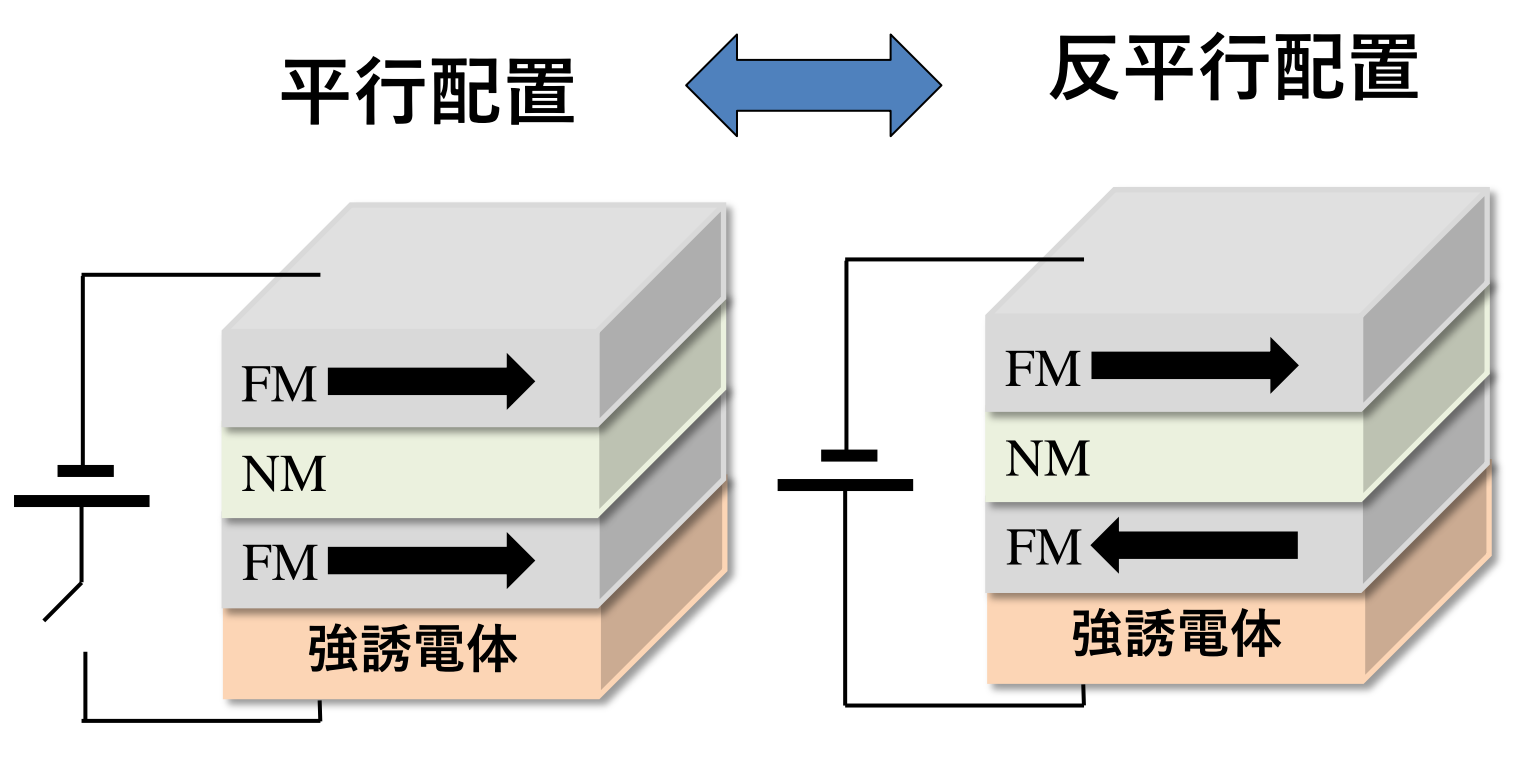
電界によって、二つの強磁性体の磁化の相対位置を、平行⇔反平行と切り替える。
